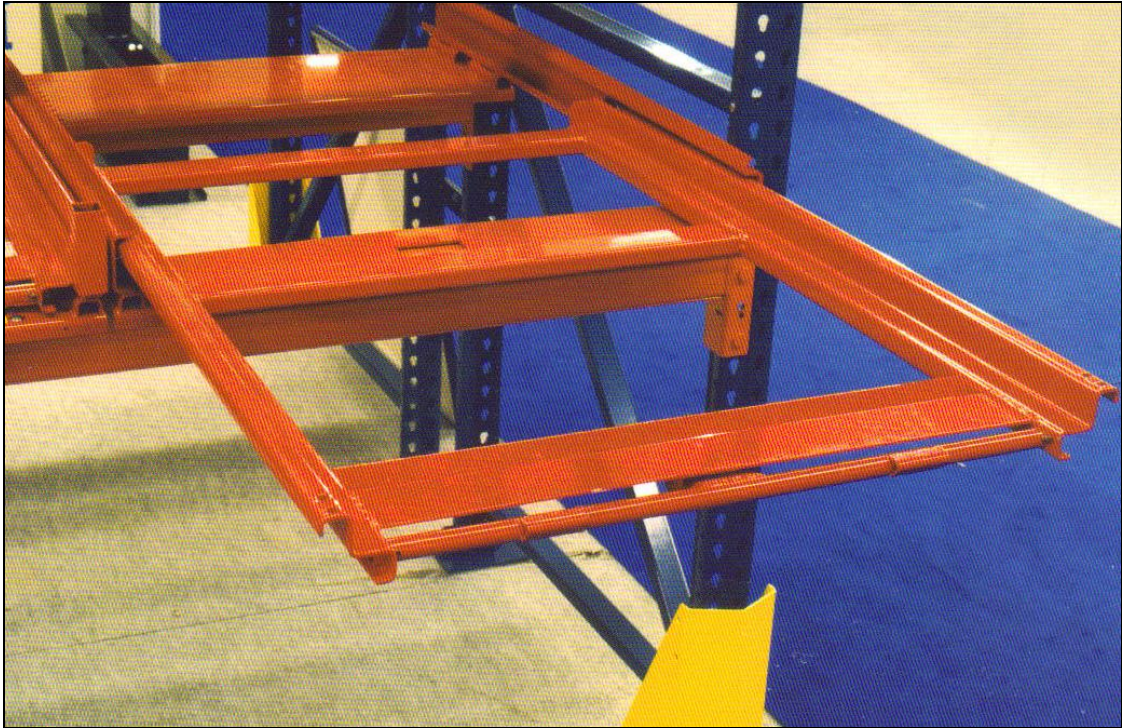
Schuiflade op het liggerniveau
